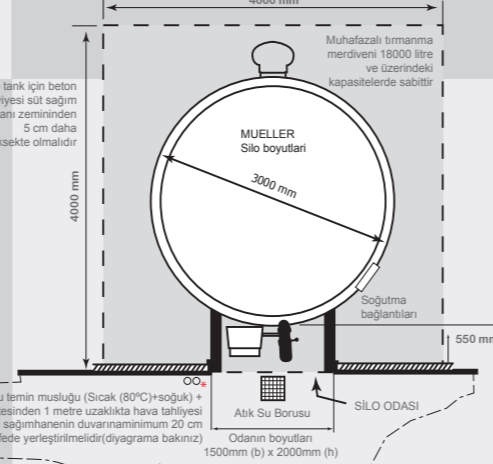
MUELLER SİLO BOYUTLARI üstten görünüm
