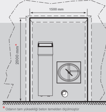
MUELLER SİLO ODASININ BOYUTLARI ön taraftan
